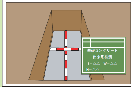
⑦基礎コンクリート 出来形検測 L=△△△ W=△△△ H=△△△
