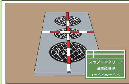
⑮上部スラブコンクリート 出来形検測 L=△△△ W=△△△
