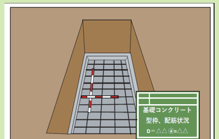
⑥基礎コンクリート 型枠、配筋状況 鉄筋 D=△△△ @=△△△
