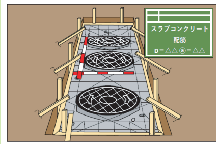
⑭上部スラブコンクリート 型枠、配筋鉄筋 D=△△△ @=△△△
