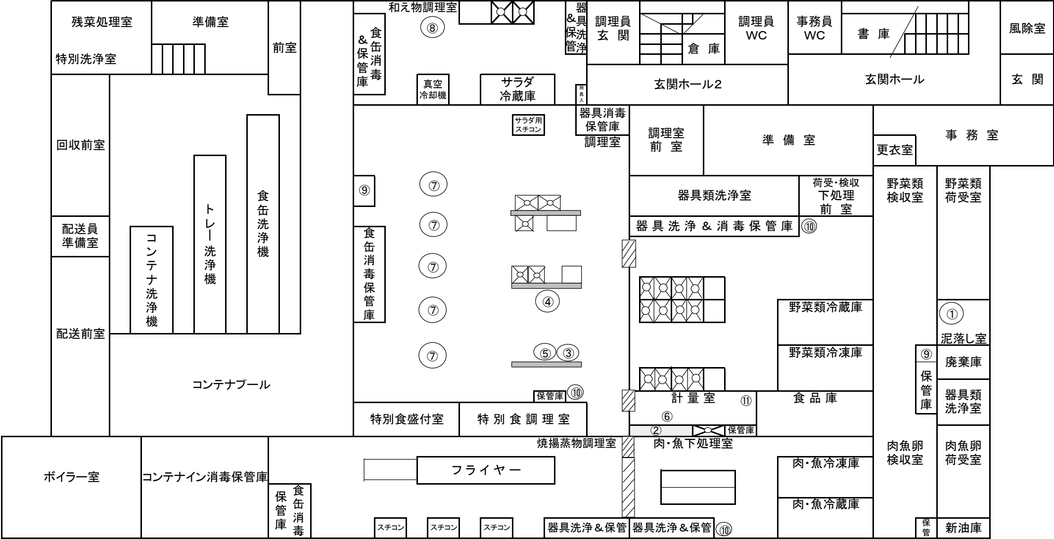
八千代町立学校給食センター主要機器等配置図
